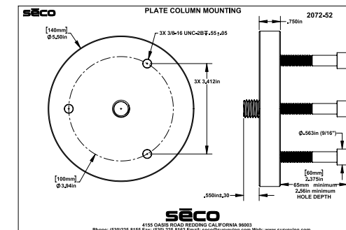
2072-52 — Column Plate
